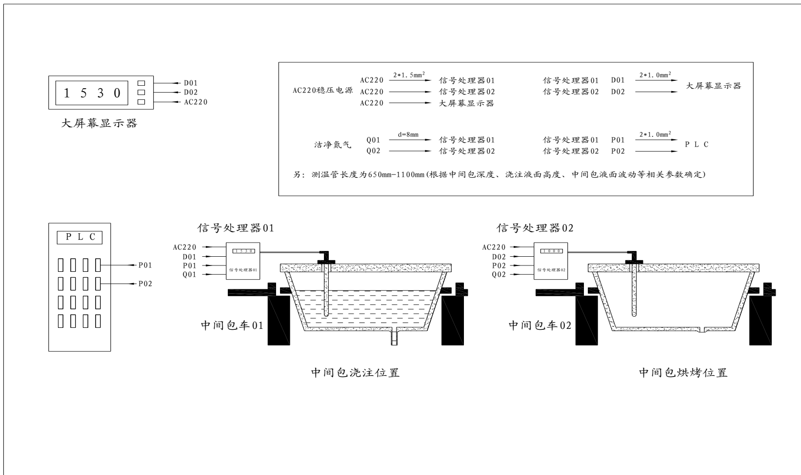
安装示意图1:
